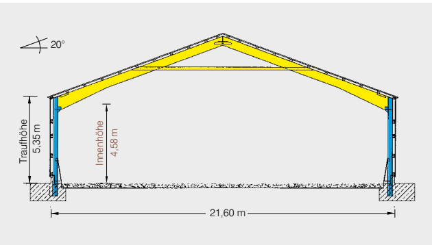
Typ RBs für freie Dachneigung
