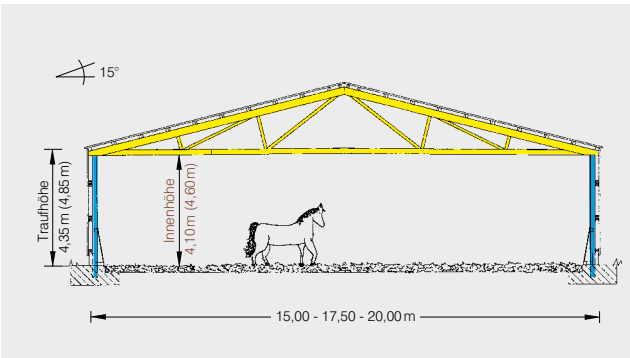
Typ FB Bewegungshalle für Pferde
