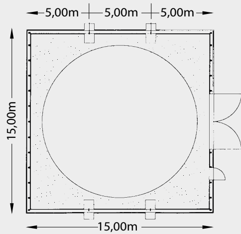
LONGIERHALLE MIT 8-ECKIGER REITBANDE
